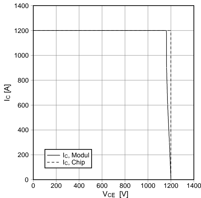
Sicherer Rückwärts-Arbeitsbereich IGBT-Wr. (RBSOA) reverse bias safe operating area IGBT-inv. (RBSOA) I_C = f(V_{CE}) V_{GE} = \pm 15\text{ V} , R_{Goff} = 3\ \Omega , T_{vj} = 125^\circ\text{C}
